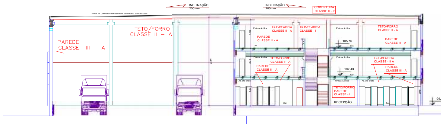
Corte AA
