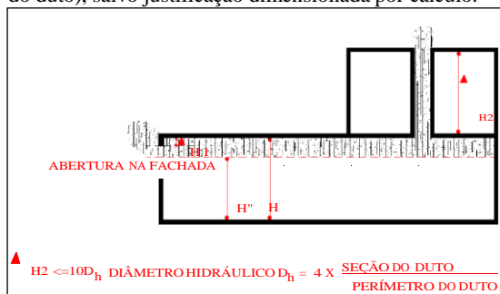
Figura 17 - Diâmetro hidráulico
