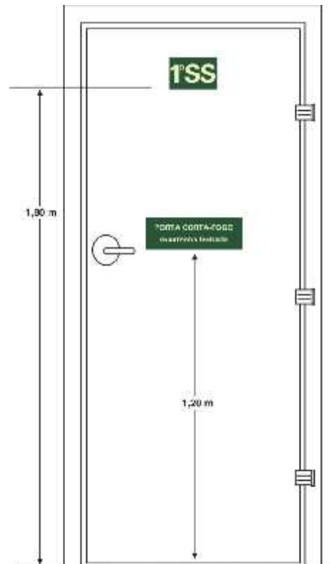
Figura C-2 - Sinalização de porta corta-fogo (vista do hall).
