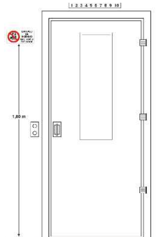
Figura C-4 - Sinalização de elevadores (vista da escada).
